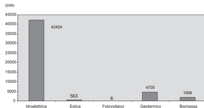
Fig. 12 - Produzione di energia rinnovabile in Italia anno 2000 (fonte ENEL)
