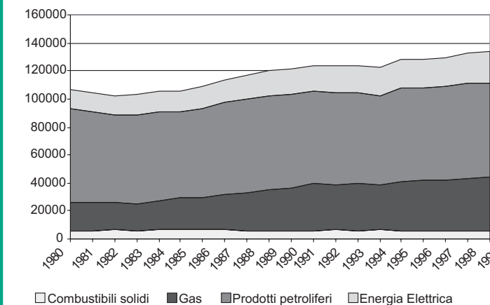
Fig.11 - Usi finali di energia per fonte (migliaia di tep)
