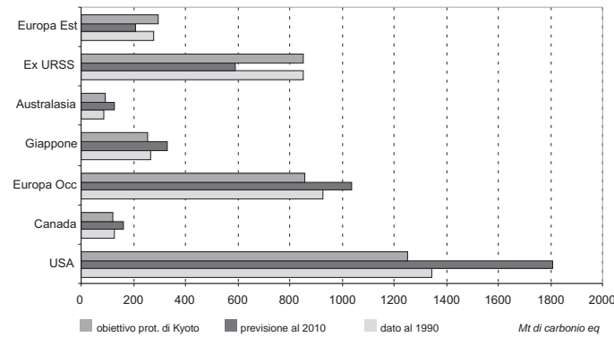
Fig. 1 - Emissioni di CO 2 : previsione IEA al 2010 (WEO 2001)
